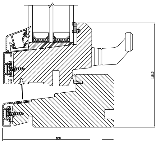
Vridfönster med aluminiumbeklädnad - vertikalt snitt
