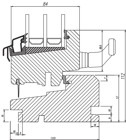
Vridfönster - vertikalt snitt
