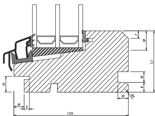
Karmfast fönster - vertikalt snitt
