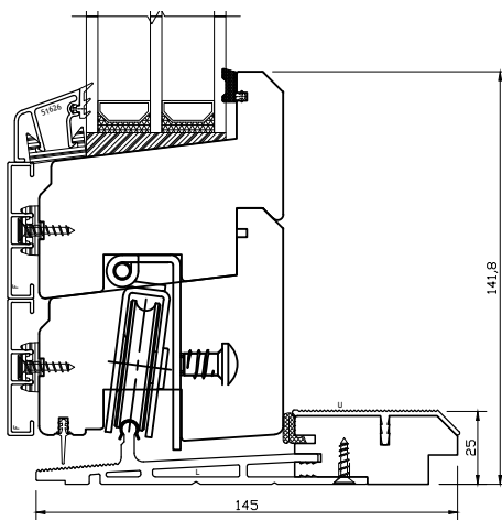
Skjutparti med aluminiumbeklädnad - vertikalt snitt
