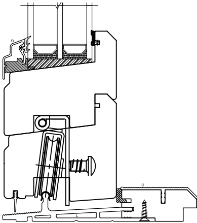
Skjutparti - vertikalt snitt
